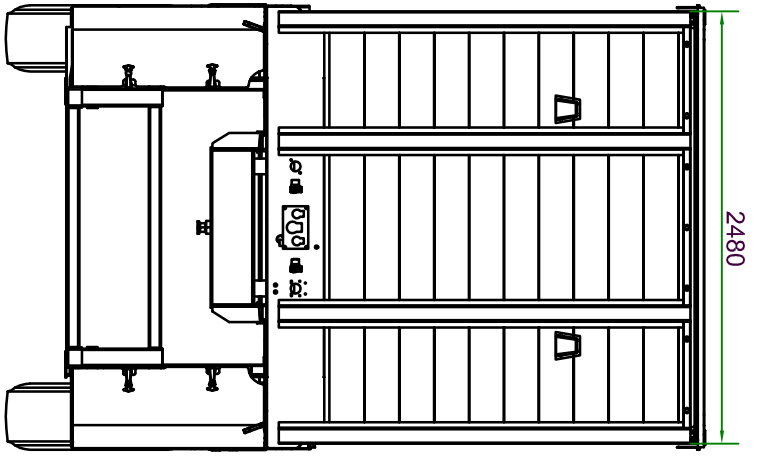
A (1 : 30)
